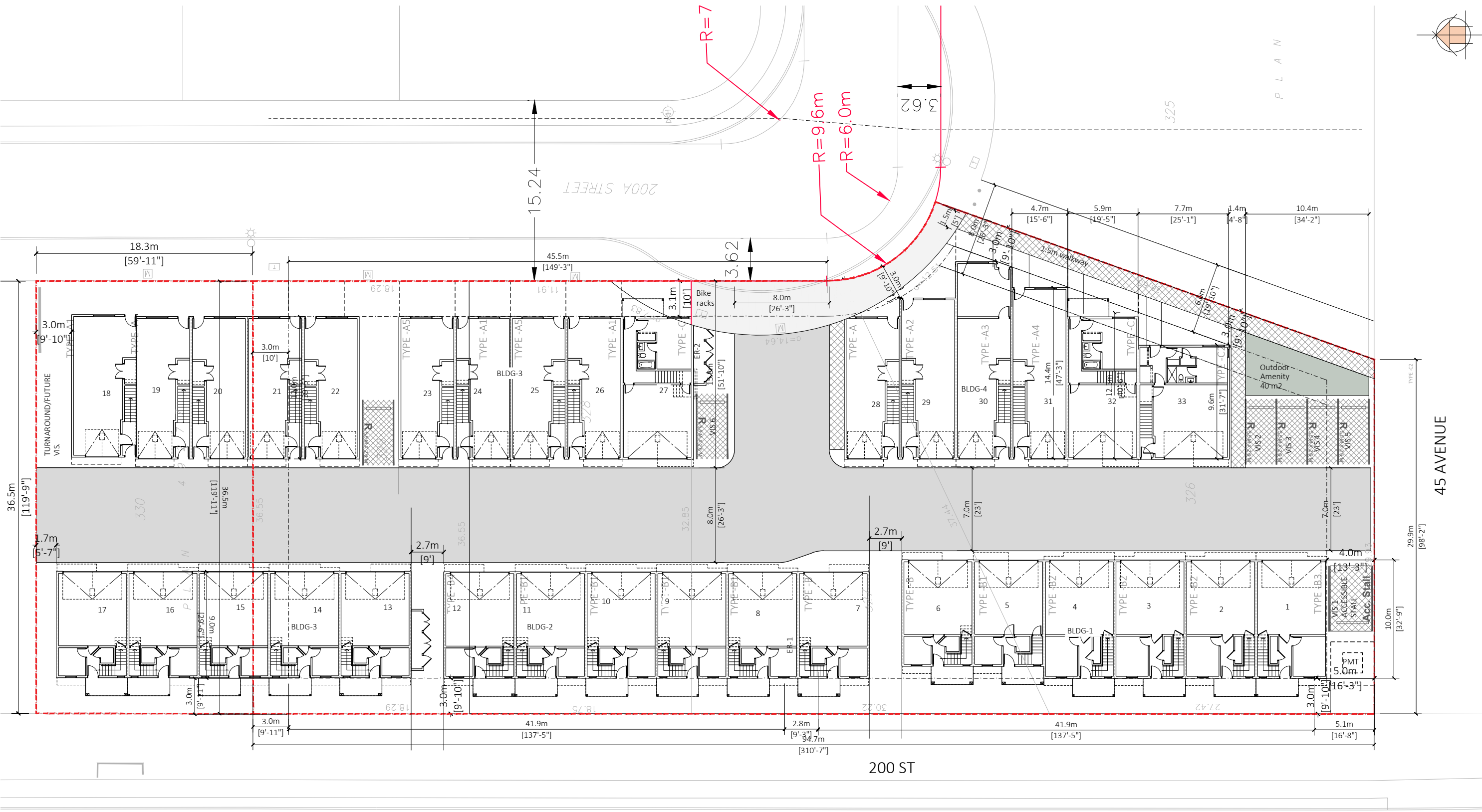
1 SITE PLAN n.t.s
