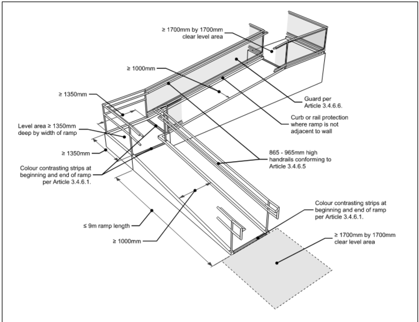
3.8.3.5. Ramp Design
